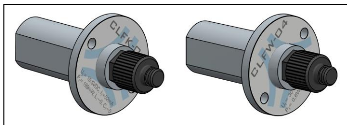
Rys. 21a Nadajniki wymienne
