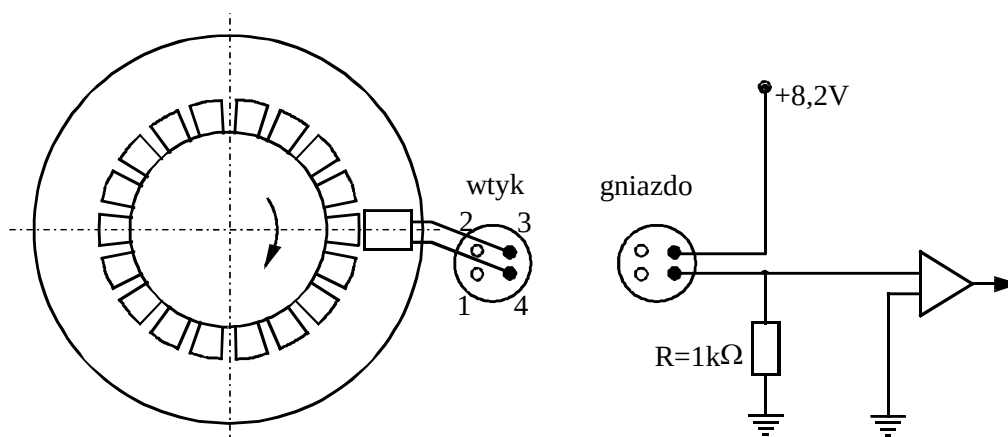
Rys.5. Schemat przyłączenia nadajnika HF
