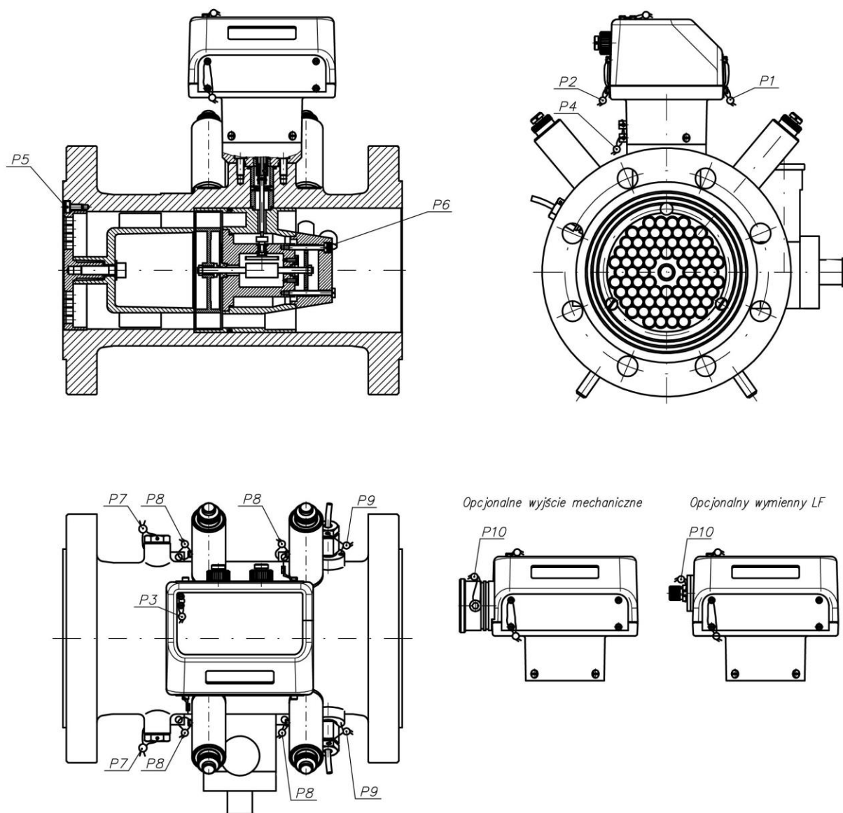
Rys. 13a. Punkty umieszczania plomb na gazomierzach CGT-02 (wersja 1)
