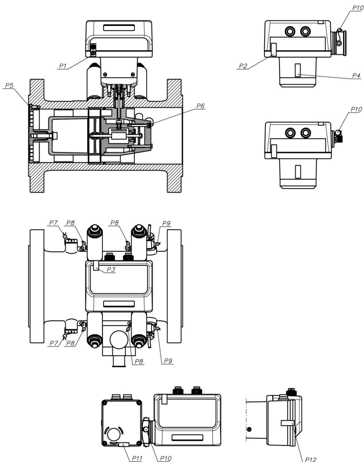
Rys. 13b. Punkty umieszczania plomb na gazomierzach CGT-02 (wersja 2)
