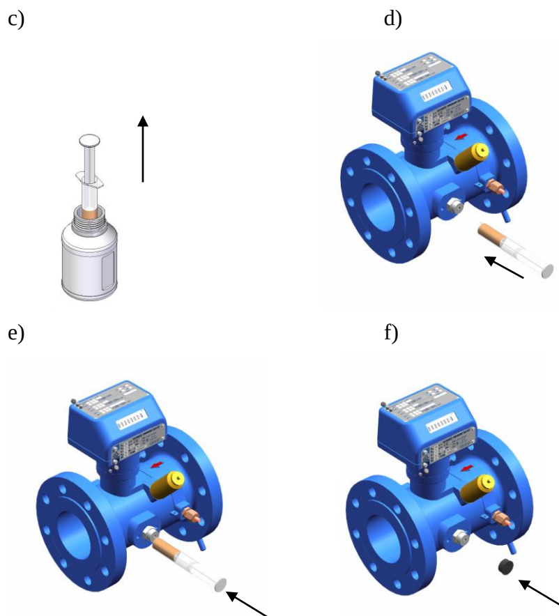
Rys. 20 Czynności podczas smarowania gazomierza z zaworem zwrotnym
