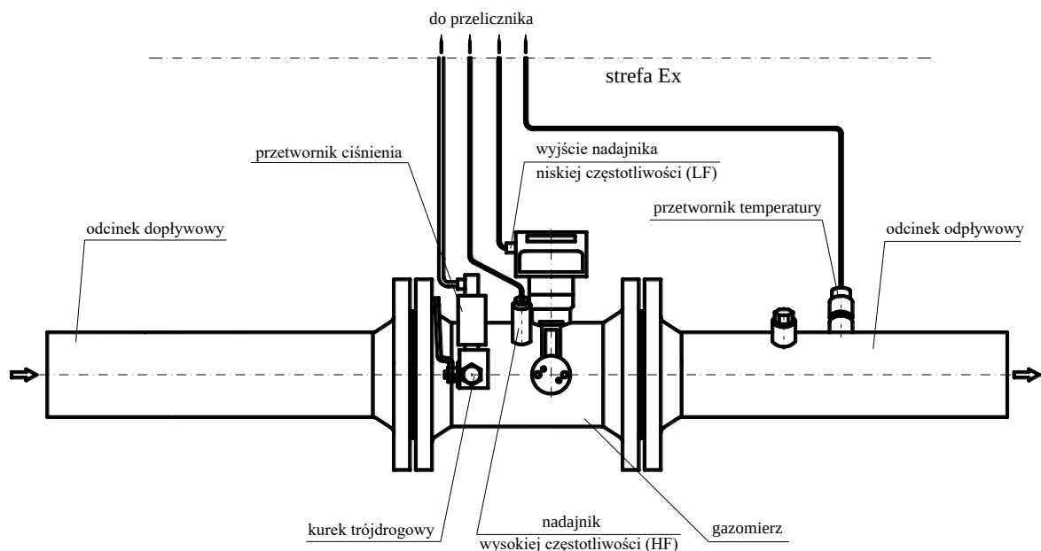
Rys. 25. Układ przyłączeń zespołu korekcyjnego umieszczonego poza strefą zagrożoną wybuchem (strefą Ex) zasilanego z sieci 220 V
