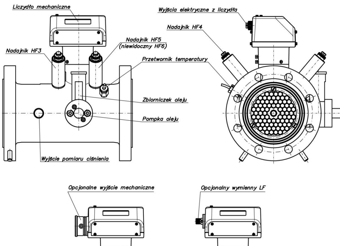
Rys.3. Usytuowanie wyjść pomiarowych w gazomierzach CGT-02
