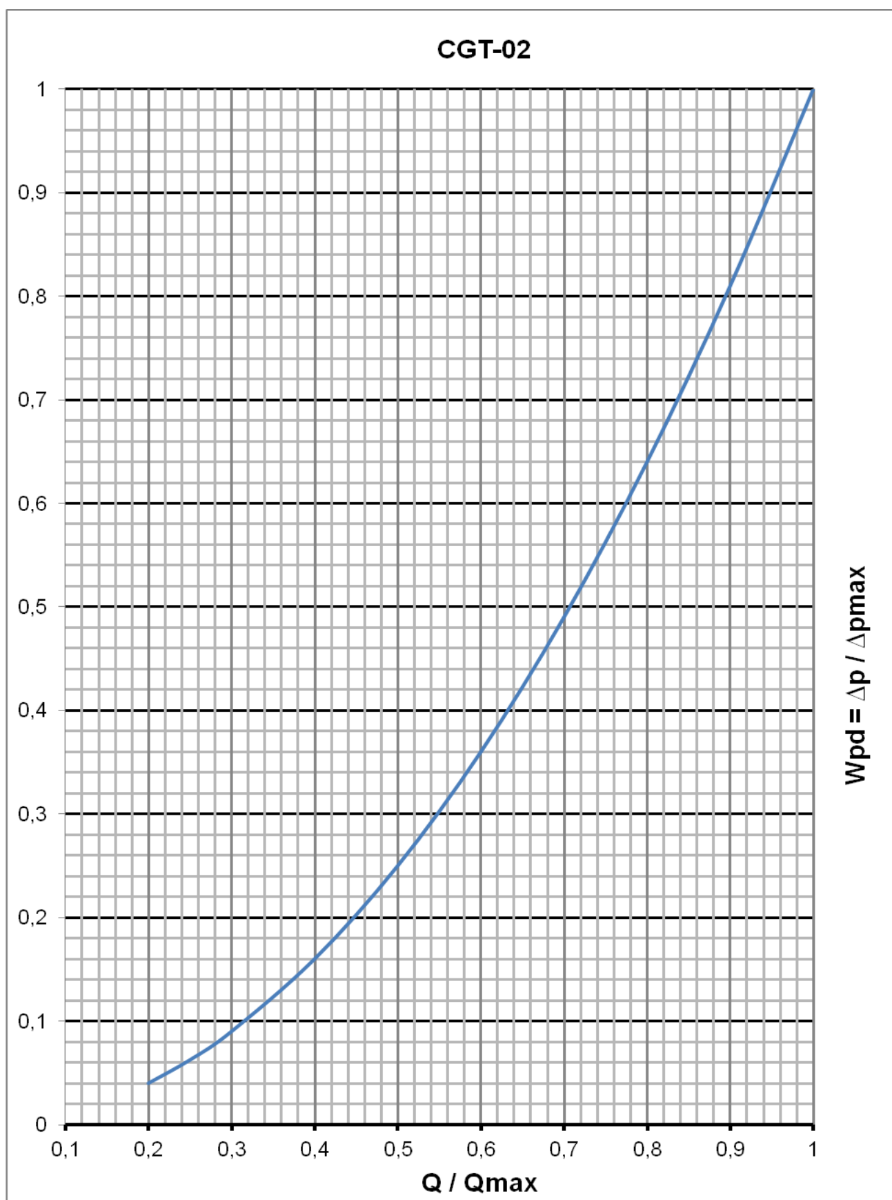
Rys.1. Współczynnik straty ciśnienia W_{pd} w funkcji strumienia względnego Q/Q_{\max}
