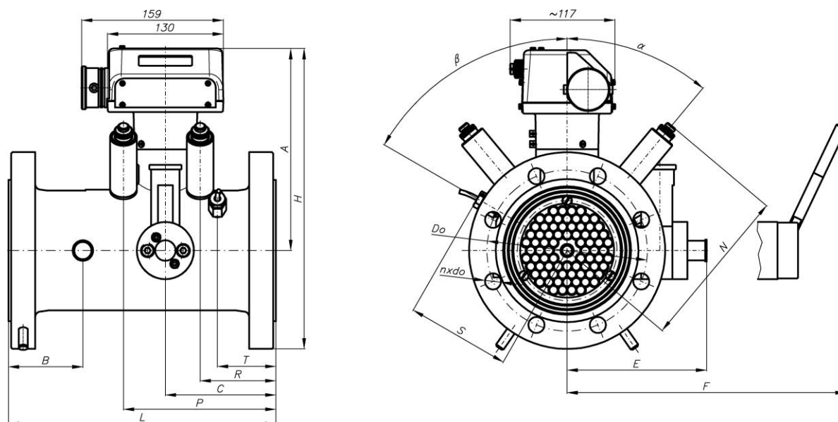
Rys.18. Podstawowe wymiary gazomierzy turbinowych CGT-02.
