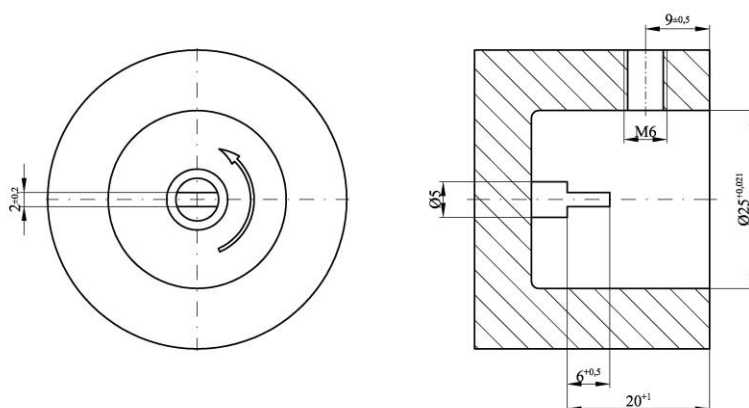
Rys. 8a Napędowy wałek wyjścia mechanicznego
