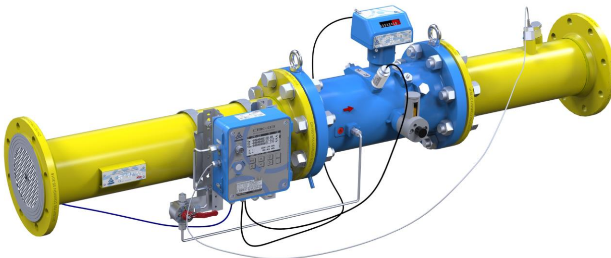
Rys. 24. Zestaw montażowy gazomierza turbinowego CGT-02 z przelicznikiem CMK-03 (przelicznik mocowany na odcinku dopływowym)
