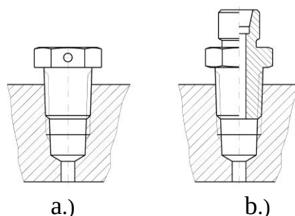
Rys 6. Gniazdo pomiaru ciśnienia \frac{1}{4}\text{NPT}
