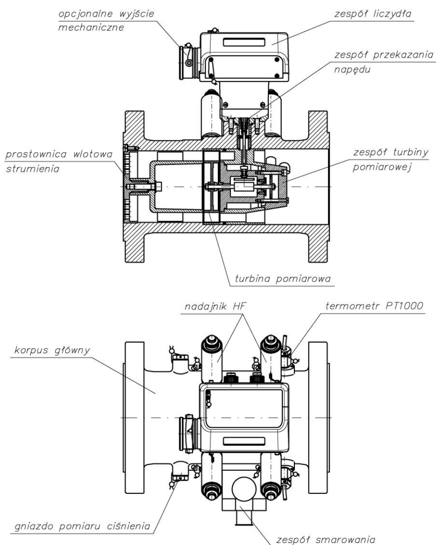
Rys.2. Gazomierz turbinowy CGT-02 w przekroju
